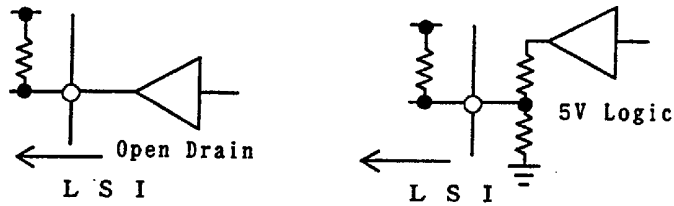
Input Pin
