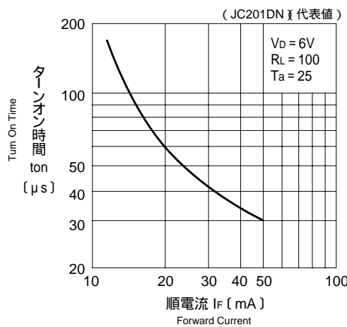
ターンオン時間 - 順電流特性
