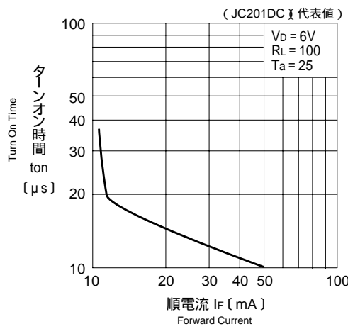
ターンオン時間 - 順電流特性
