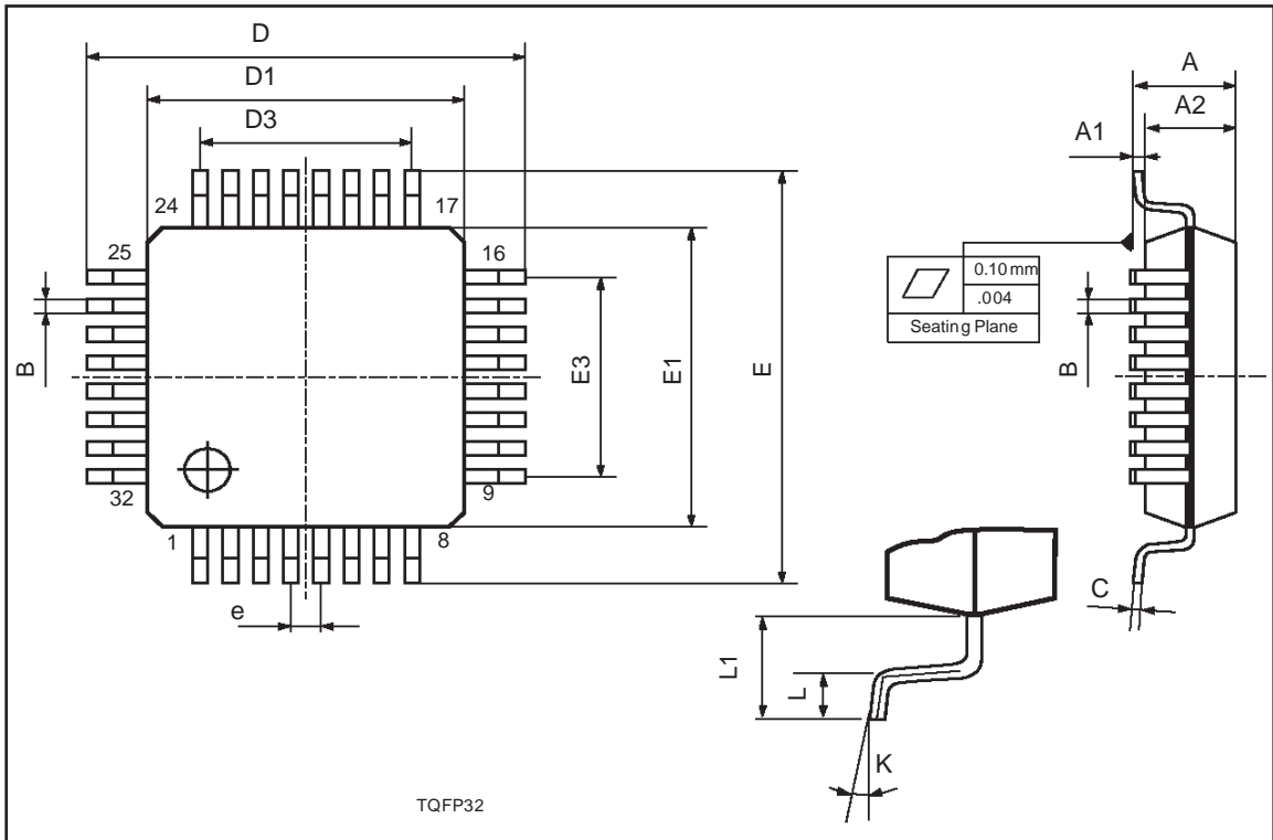
TQFP32
