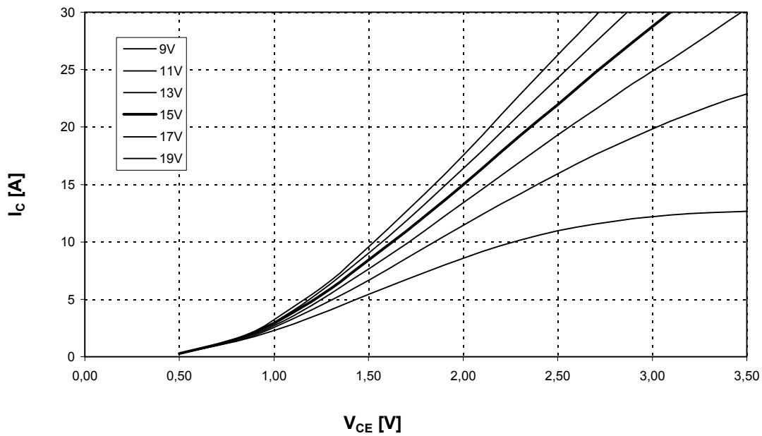
Ausgangskennlinienfeld Wechsler. (typisch) Output characteristic Inverter (typical)
