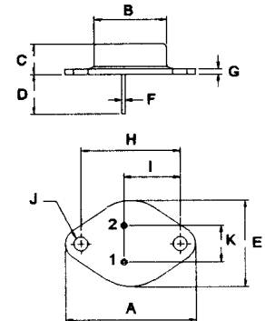
TO-3
