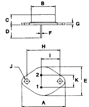
TO-3
