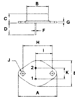
TO-3
