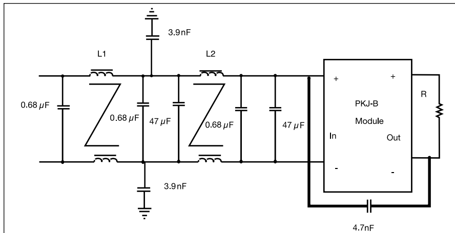
L1=L2=574µH
