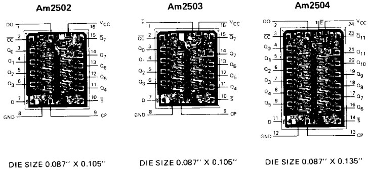
DIE SIZE 0.087" X 0.105"
