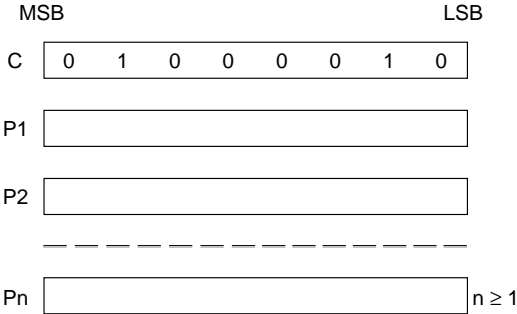
Figure 24. MWRITE parameters
