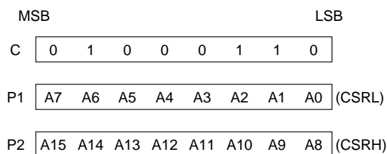
Figure 22. CSRW parameters
