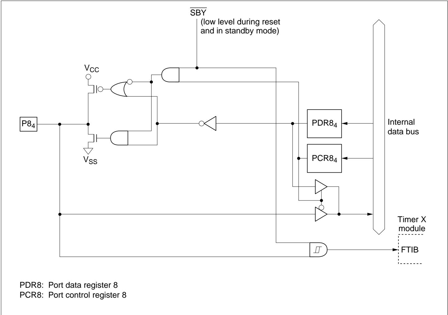
Figure C.7 (d) Port 8 Block Diagram (Pin P8 4 )
