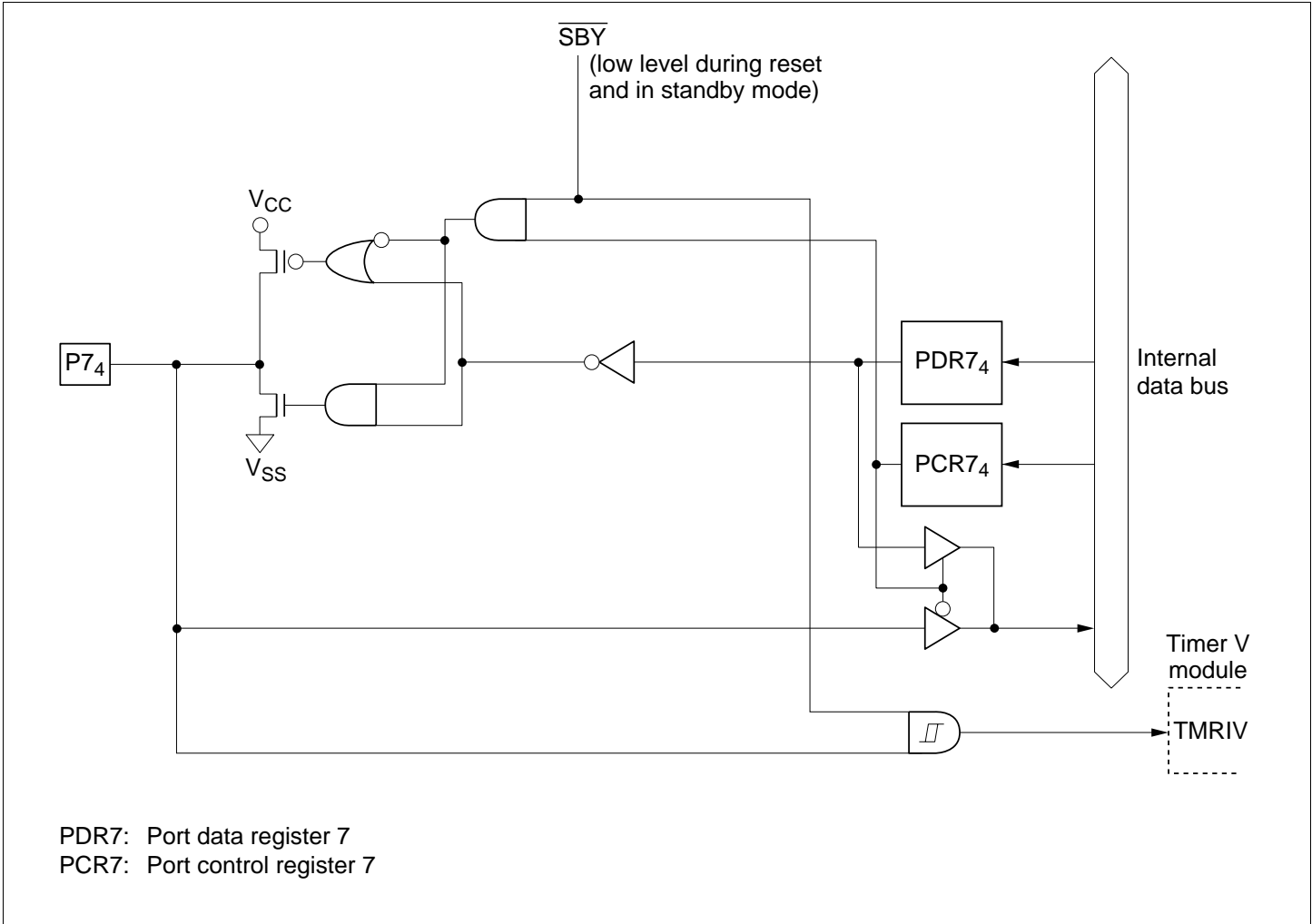
Figure C.6 (d) Port 7 Block Diagram (Pin P7 4 )
