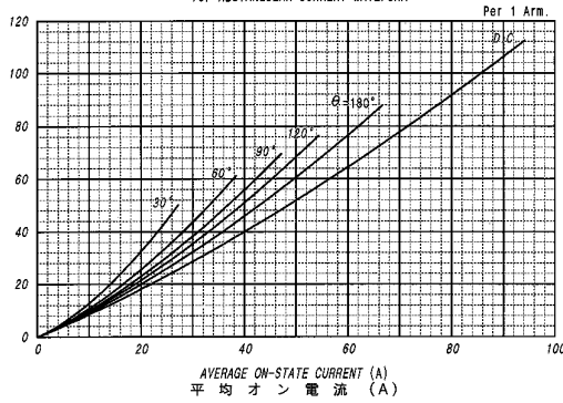
平均オン電力損失特性 AVERAGE ON-STATE POWER DISSIPATION
