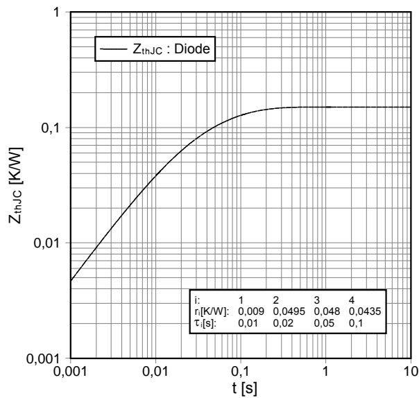
Transienter Wärmewiderstand Diode-Wechselr. transient thermal impedance diode-inverter
