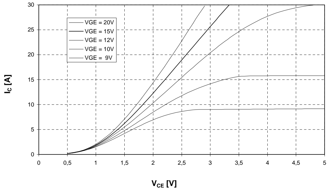
Ausgangskennlinienfeld Wechselr. (typisch) d = f(V_{CE}) Output characteristic Inverter (typical) T_{vj} = 125^\circ\text{C}
