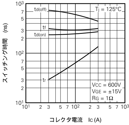
ハーフブリッジ - スwitchング特性 (代表例)
