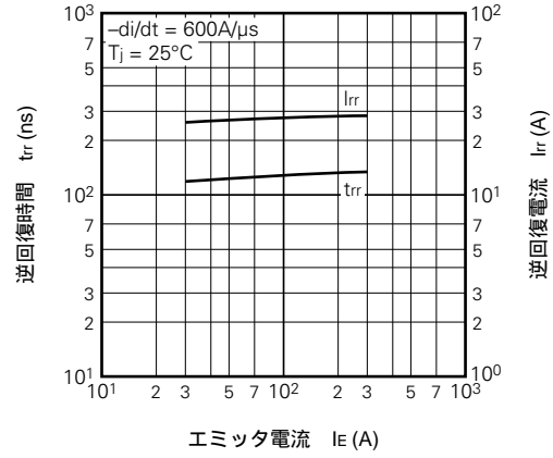
ダイオード部逆回復特性 (代表例)
