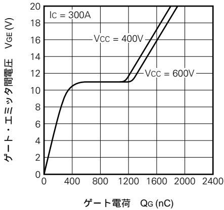
VGE - ゲート電荷 (代表例)
