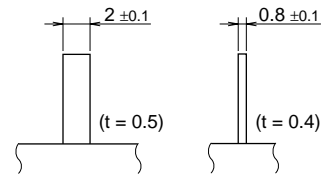
A : DETAIL
