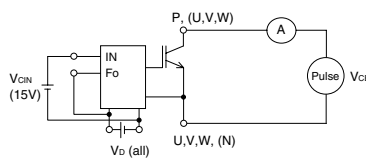
Fig. 5 I_{CES} Test
