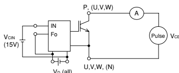
Fig. 5 I_{CES} Test
