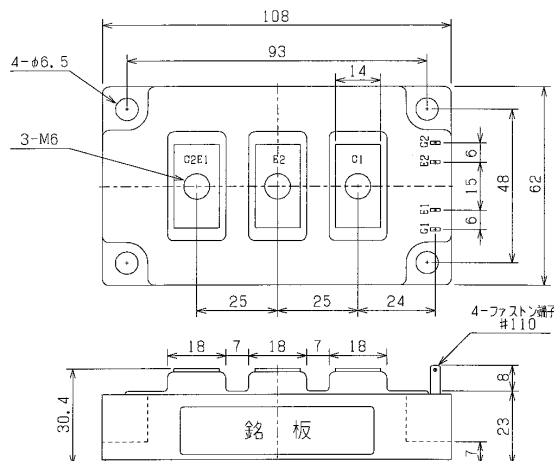
外形寸法図 OUTLINE DRAWING (単位 Dimension : mm)
