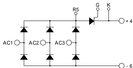
回路図 CIRCUIT
