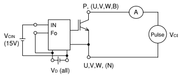
Fig. 4 I_{CES} Test
