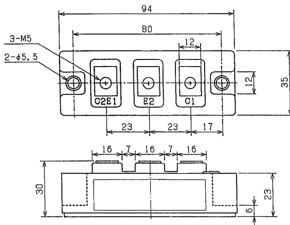
外形寸法図 OUTLINE DRAWING (単位 Dimension : mm)
