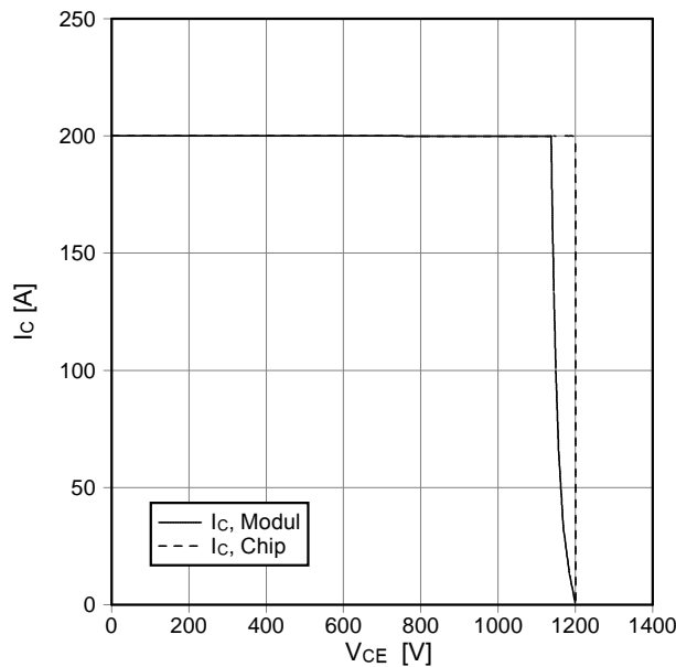
Sicherer Rückwärts-Arbeitsbereich IGBT-Wr. (RBSOA) reverse bias safe operating area IGBT-inv. (RBSOA) I_c = f(V_{CE}) V_{GE} = \pm 15\text{ V} , R_{Goff} = 3,9\ \Omega , T_{vj} = 125^\circ\text{C}
