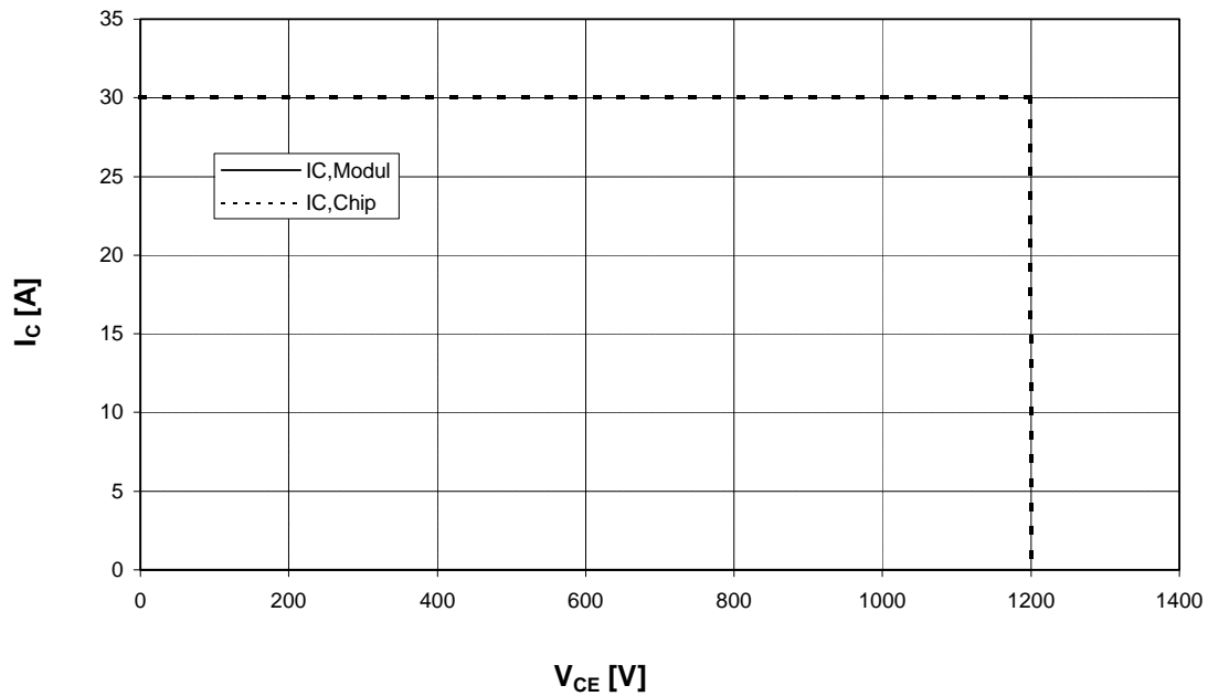
Sicherer Arbeitsbereich Wechselr. (RBSOA) I_C = f(V_{CE}) Reverse bias safe operating area Inverter (RBSOA) T_{vi} = 125^\circ\text{C}, V_{GE} = \pm 15\text{V}
