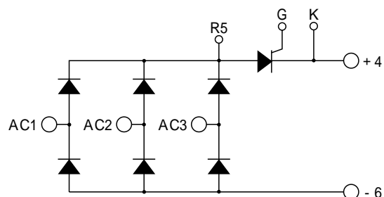
回路図 CIRCUIT
