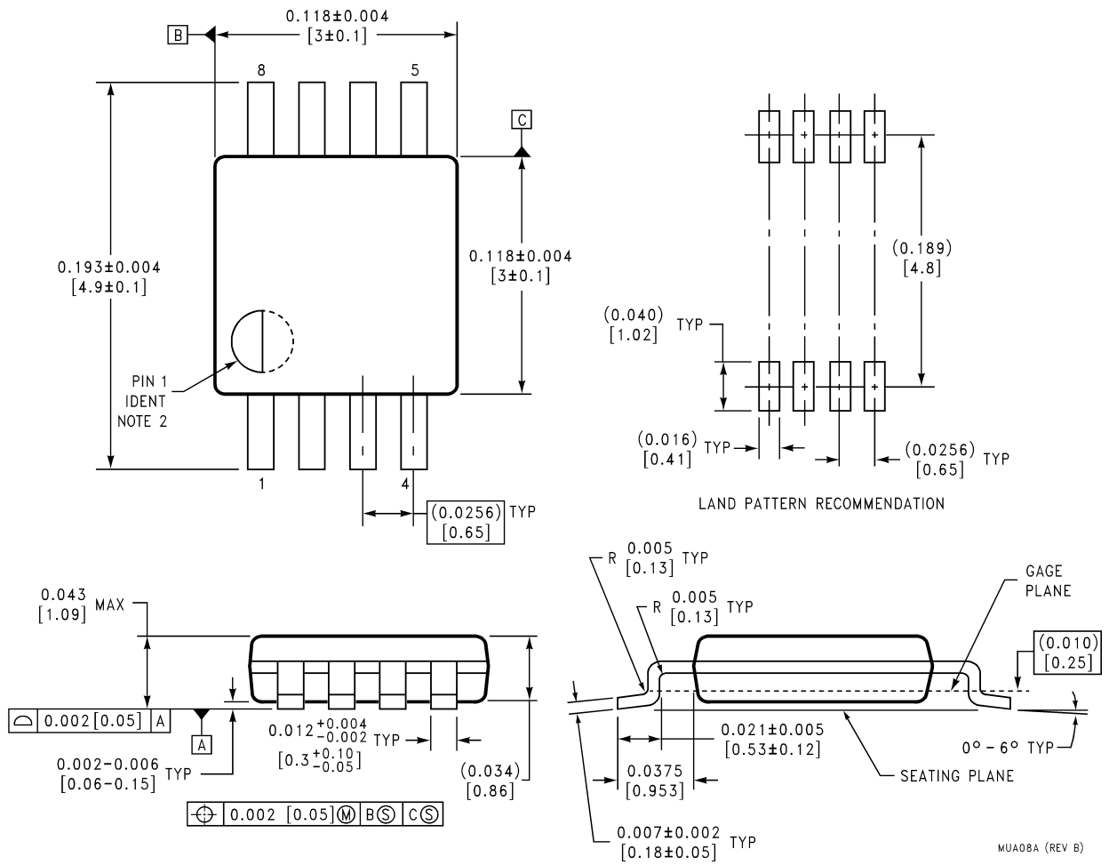
Mini SO-8 Package NS Package Number MUA08A
