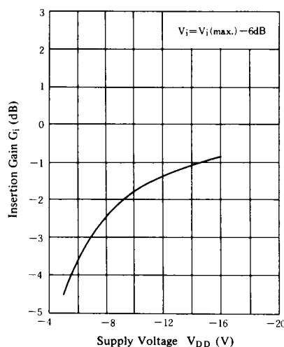
G_i - V_{DD}
