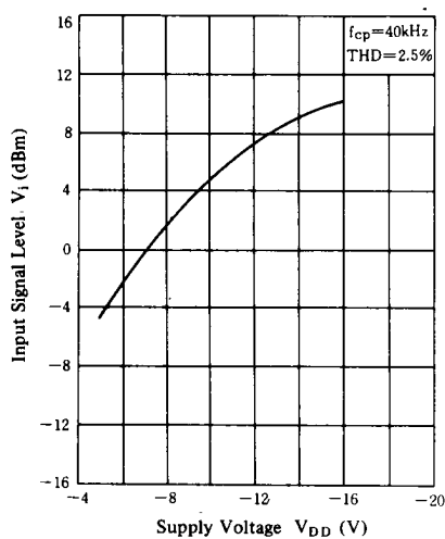
V_i - V_{DD}
