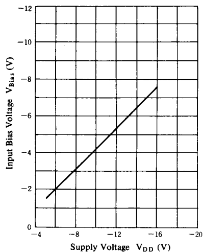
V_{Bias} - V_{DD}
