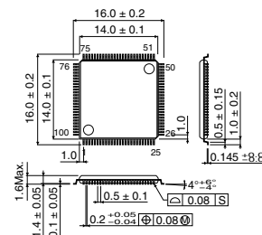
VQFP100
