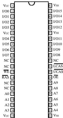
42 SOJ
