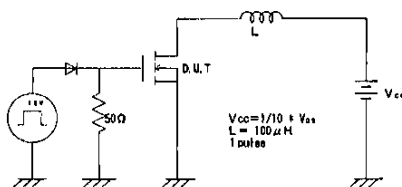
図1 測定回路 Test circuit
