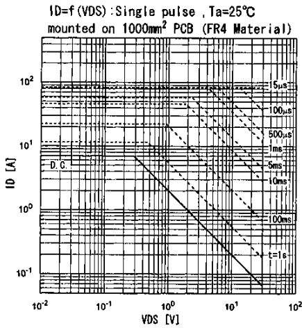
安全動作領域 Safe operating area
