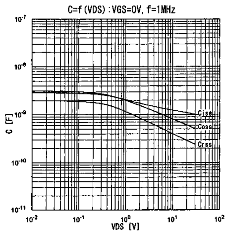
入力/出力/帰還容量 Typical capacitance
