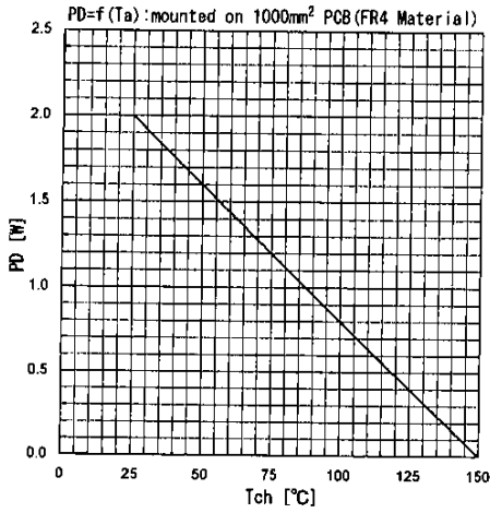
電力損失 Power dissipation
