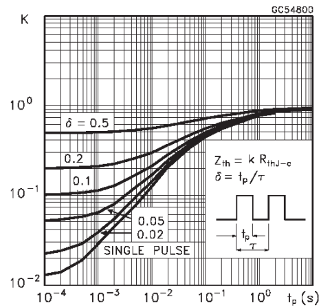
Thermal Impedance
