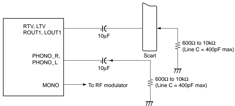
Fig. 20. Audio Output Interface
