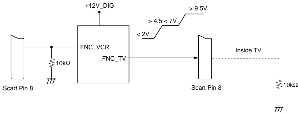
Fig. 7. TV Function Switch Output
