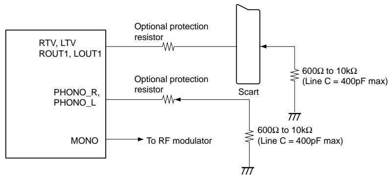
Fig. 18. Audio Output Interface
