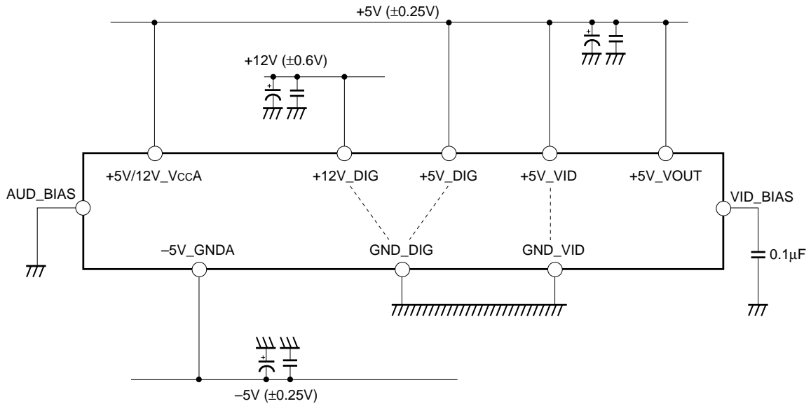
Fig. 24. Dual Supply
