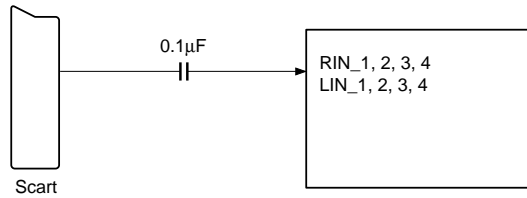
Fig. 17. Audio Input Interface
