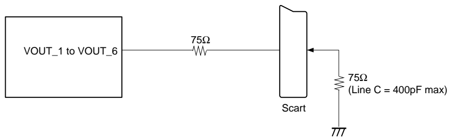
Fig. 16. Video Output Interface
