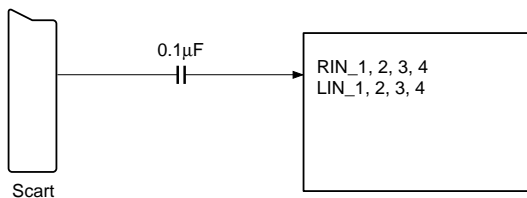
Fig. 19. Audio Input Interface
