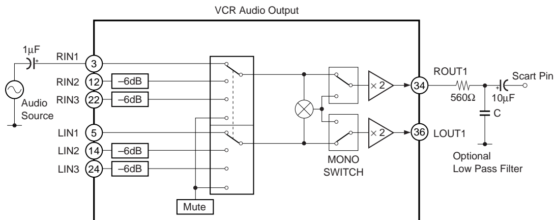
Fig. 2-2. VCR Audio Output
