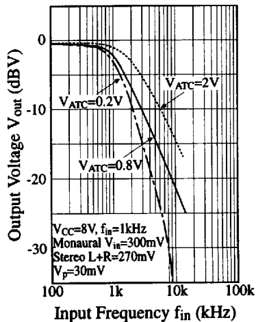
V_{out} - f_{in}
