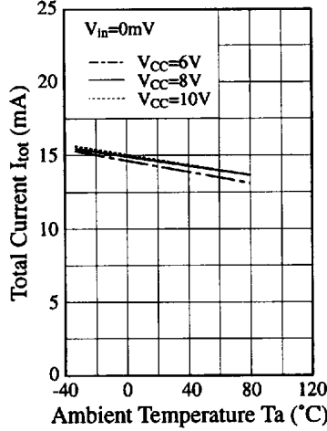
I_{tot} - T_a
