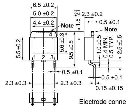
TO-252 (MP-3Z)
