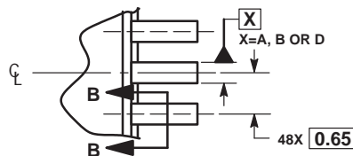
VIEW Y
