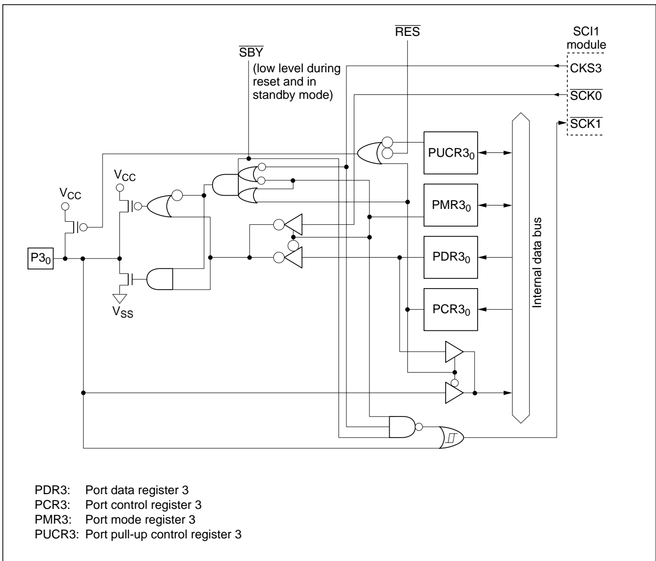
Figure C-3 (d) Port 3 Block Diagram (Pin P3 0 )
