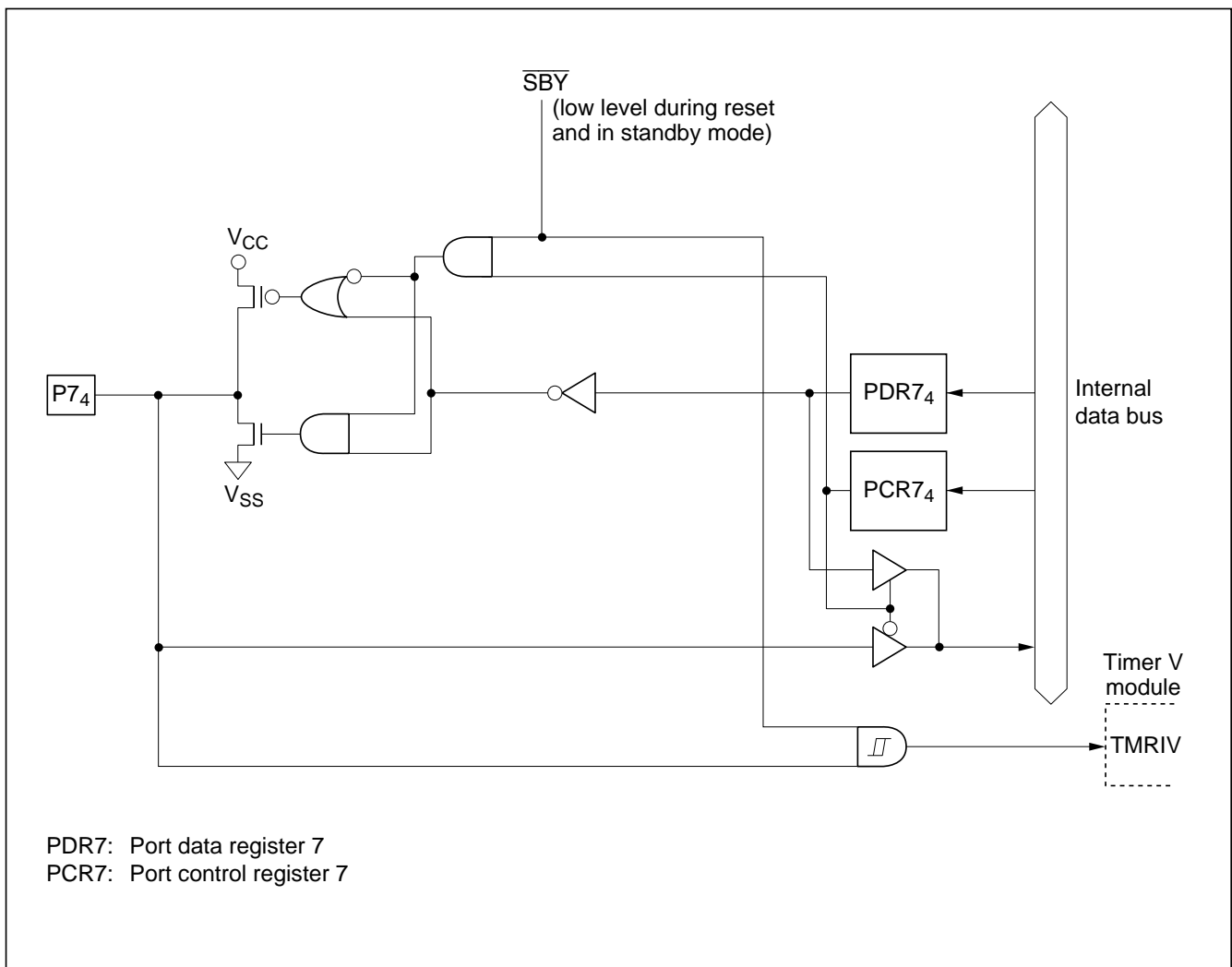
Figure C-6 (d) Port 7 Block Diagram (Pin P7 4 )
