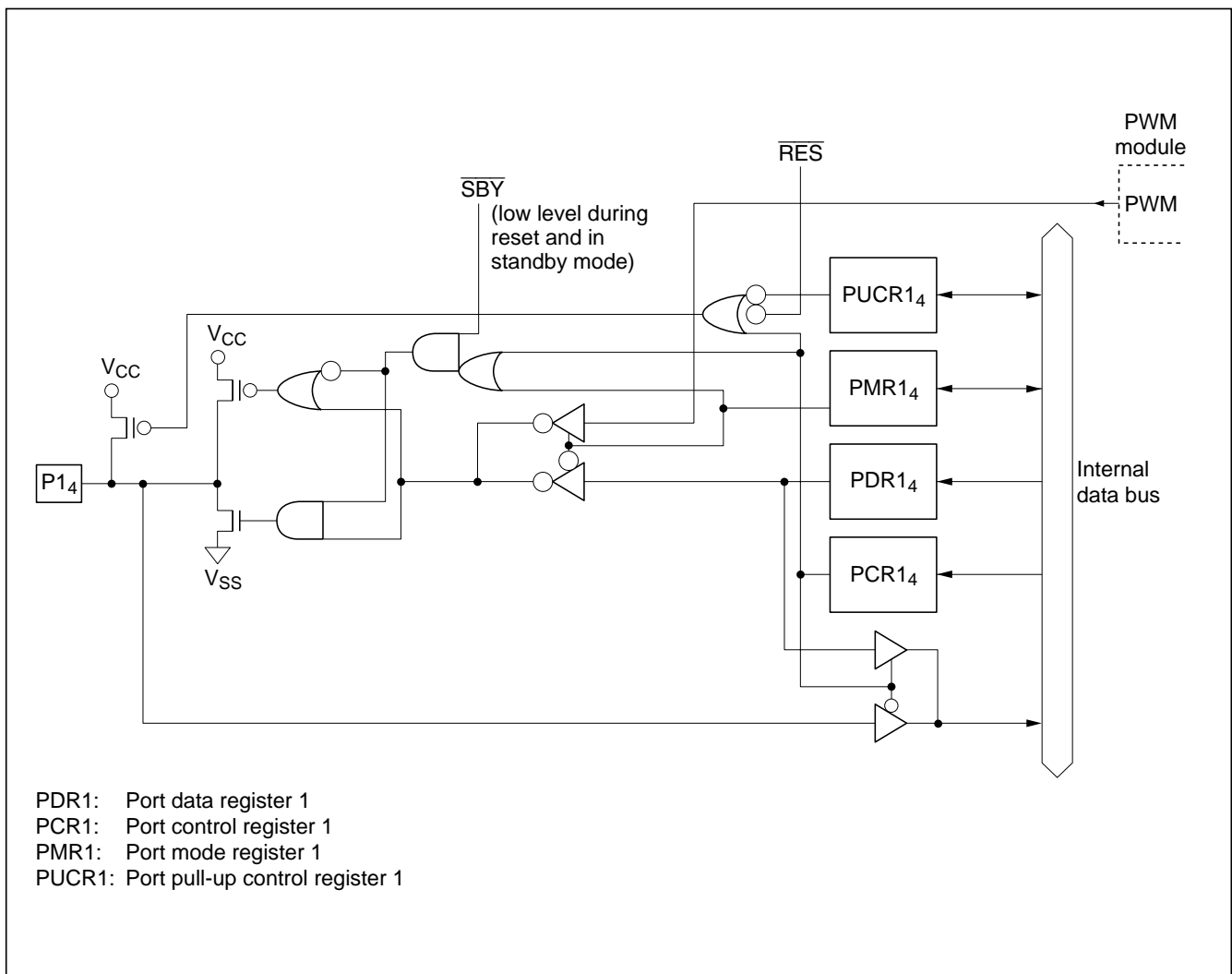
Figure C-1 (d) Port 1 Block Diagram (Pin P1 4 )
