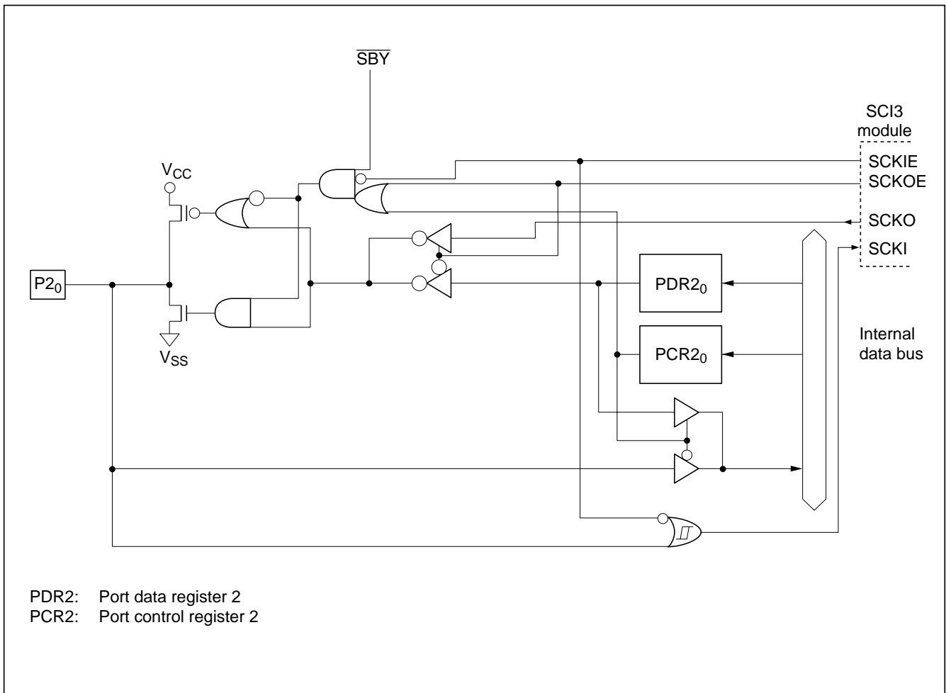
Figure C-2 (d) Port 2 Block Diagram (Pin P20)
