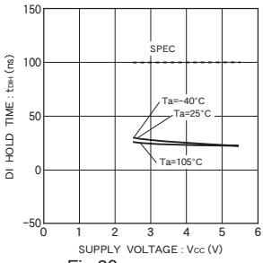
Fig.20 DI hold time t_{DIH}
