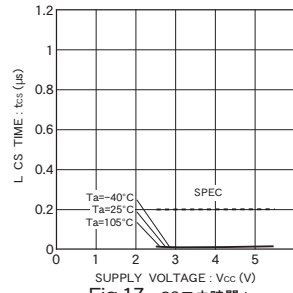
Fig.17 CS口時間 t_{cs}
