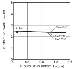
Fig. 6 H output voltage V_{OH-IOH}(V_{CC}=2.5V)
