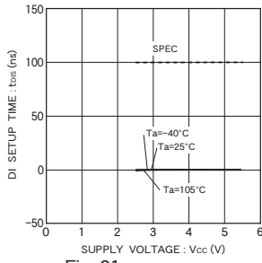
Fig. 21 DI setup time t_{DIS}
