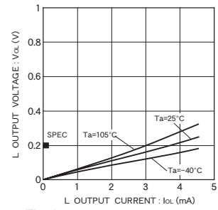
Fig. 4 L output voltage V_{OL-IOL}(V_{CC}=2.5V)
