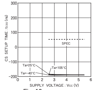
Fig. 19 CS setup time t_{cSS}
