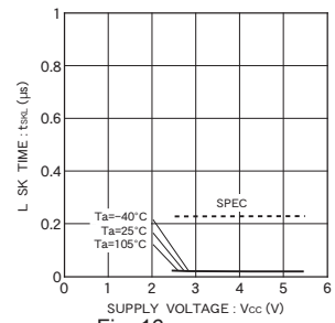
Fig. 16 SK low time t_{sKL}
