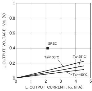
Fig. 5 L output voltage V_{OL-IOL}(V_{CC}=4.0V)
