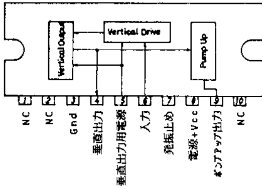
ピン接続図
