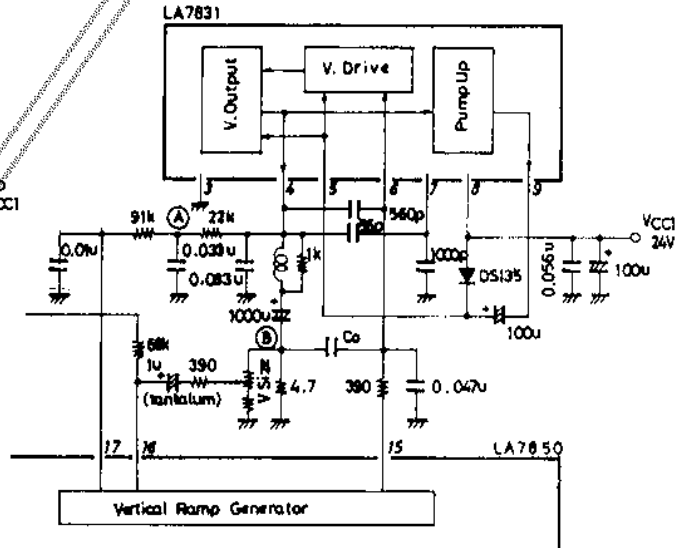
応用回路例3. LA7850の垂直出力
