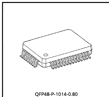
QFP48-P-1014-0.80 Weight : 1.47 g (Typ.)
