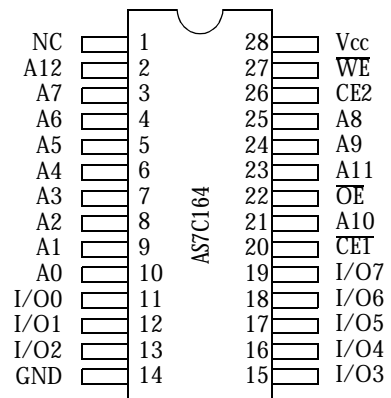
28-pin DP, SOJ (300 mL)
