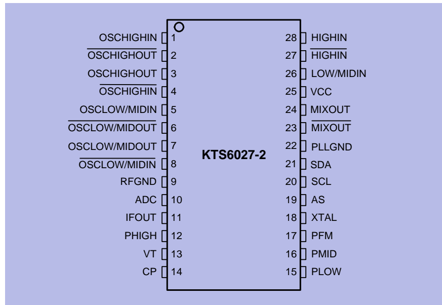
KTS6027-2_Pin_config
