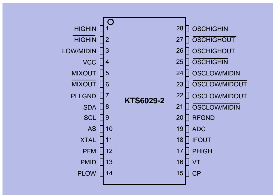
KTS6029-2_Pin_config
