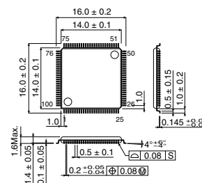
VQFP100
