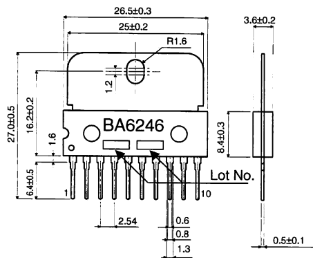
HSIP10 (Unit:mm)
