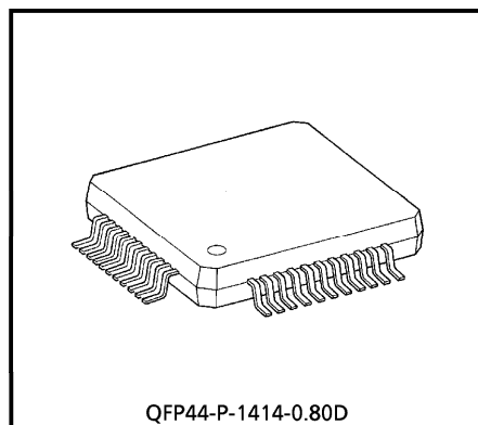
Weight : 1.07g (Typ.)
