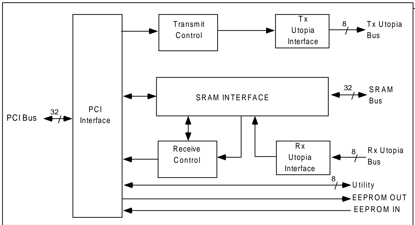
Block Diagram of the 77252 ABR SAR
