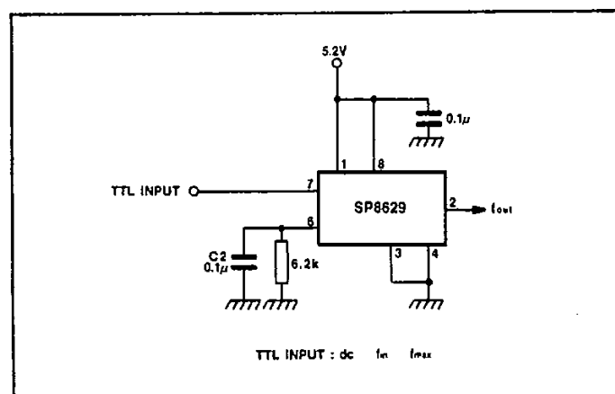
Fig.7 TTL input (DC I_{in} < I_{max} )
