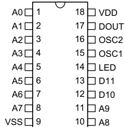
HT6012 -18 DIP-A
