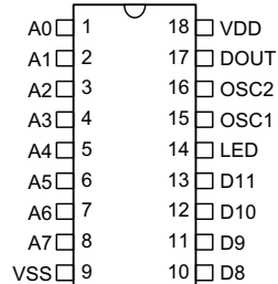
HT6014 -18 DIP-A
