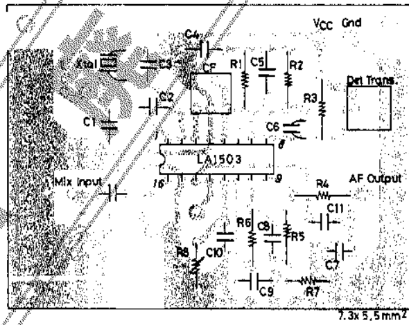
プリントパターン例 (銅箔面側)
