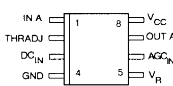
8 PIN SOIC
